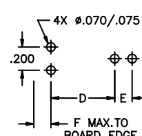
P.C. LAYOUT
